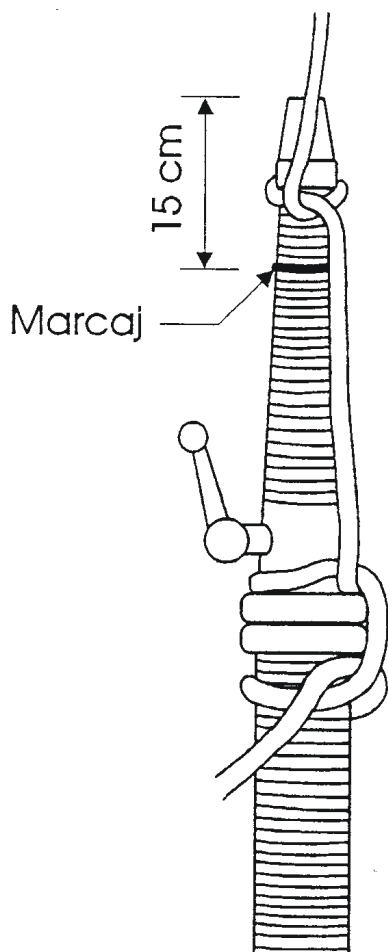
FIGURA c - FIXAREA ȚEVII CU CORDIȚA
